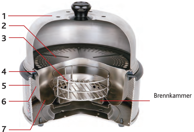
4 Gummiabstandshalter 5 Außenschale
